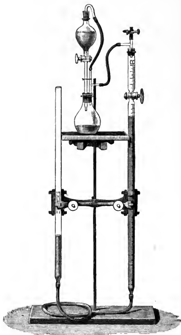
Fig. 7.—NITROGEN-EVOLUTION APPARATUS.
